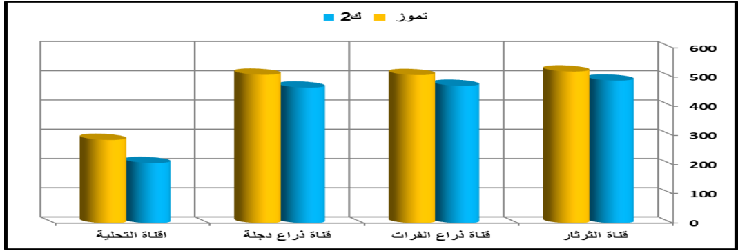
شكل (٥) قيم العسرة الكلية الشهرية للقناة الثرثار للعام ٢٠٢٢
